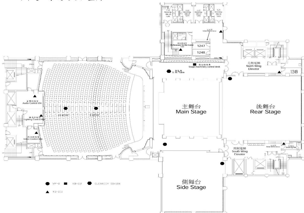
SD-2-2 內部通話系統迴路位置圖
