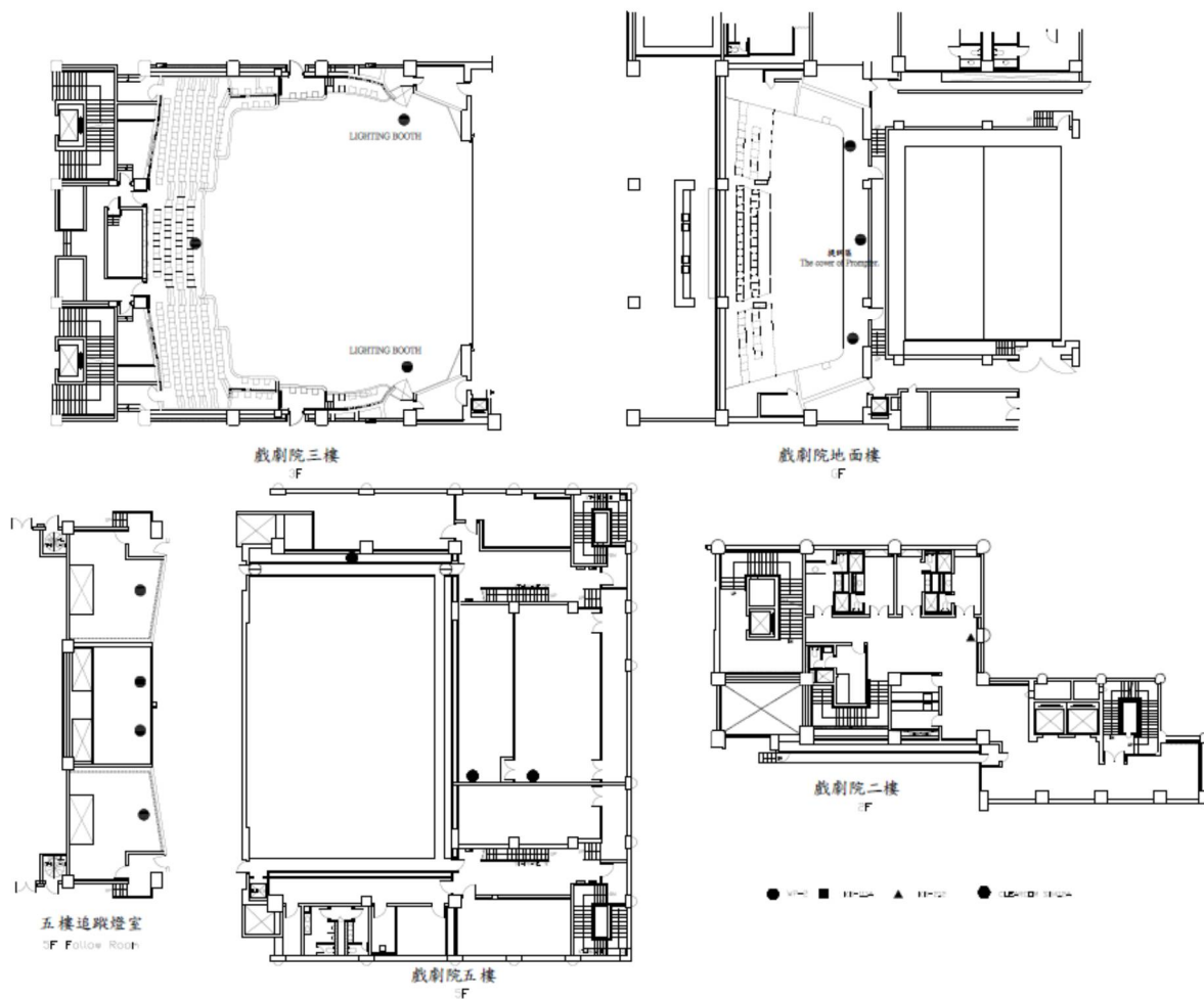
SD-2-2 內部通話系統迴路位置圖
